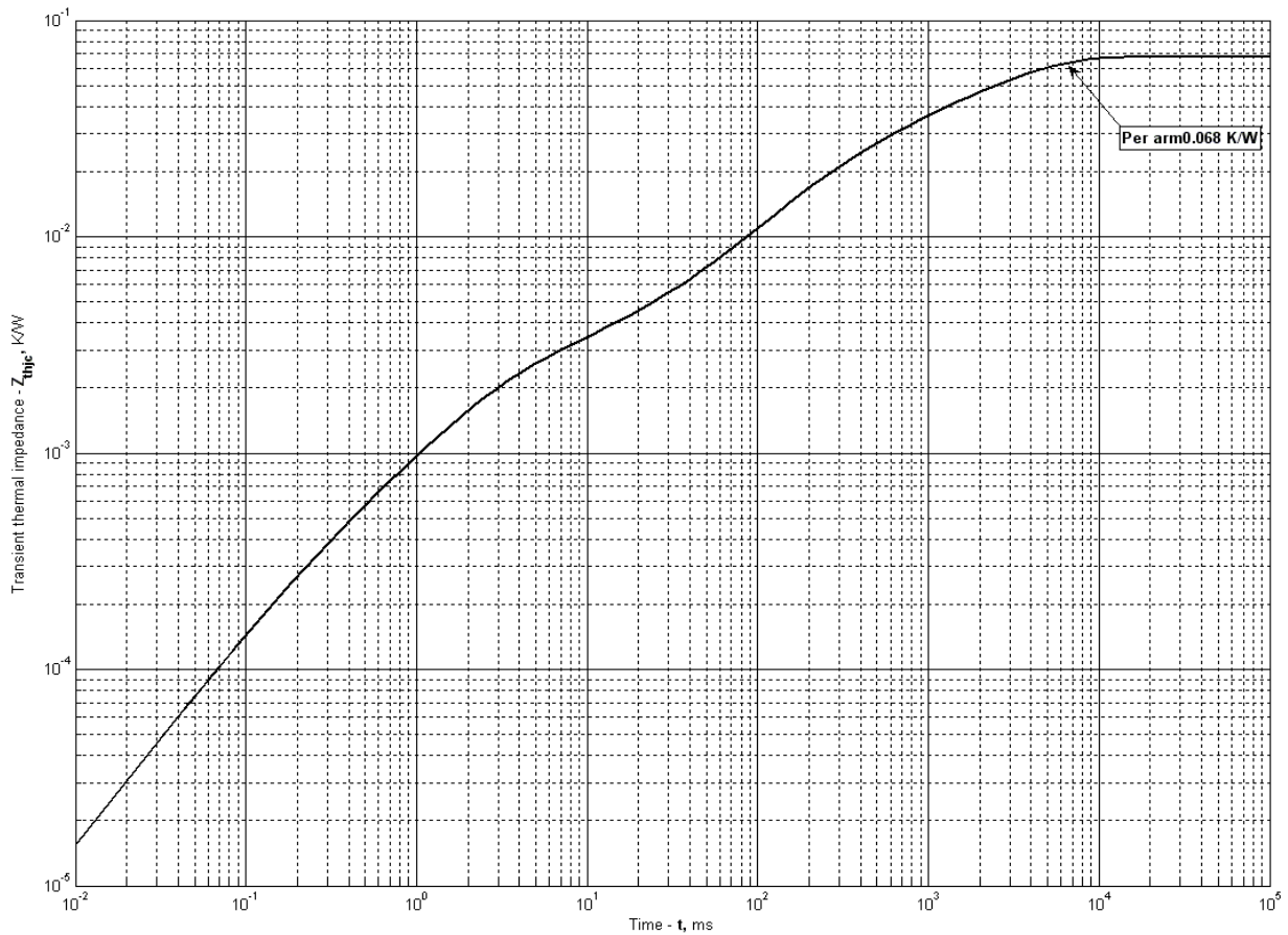
Fig 2 – Transient thermal impedance per arm (AC)
